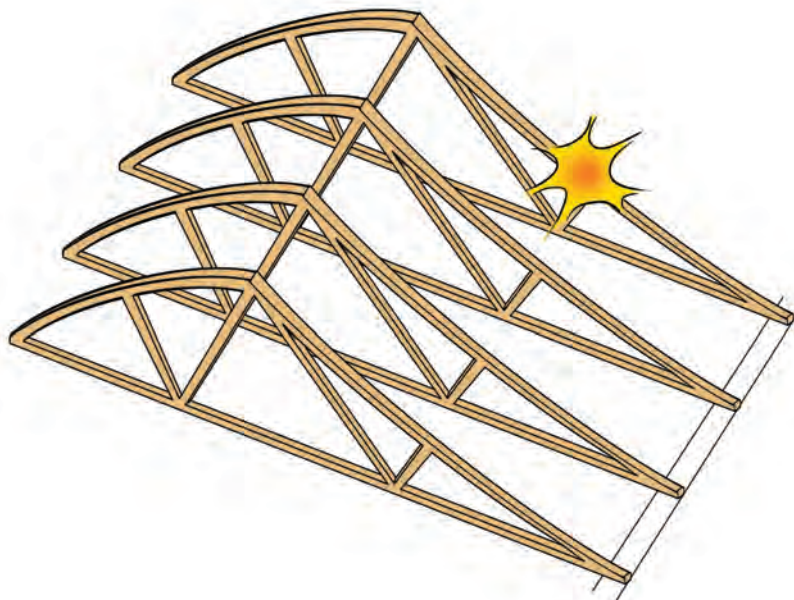
Figure 2.2. Le flambement d'un groupe de fermes peut entraîner des désordres sur la charpente
