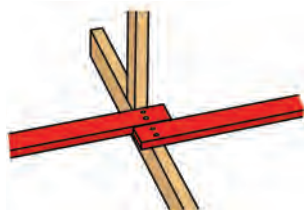
Figure 2.7. Fixation des barres filantes
