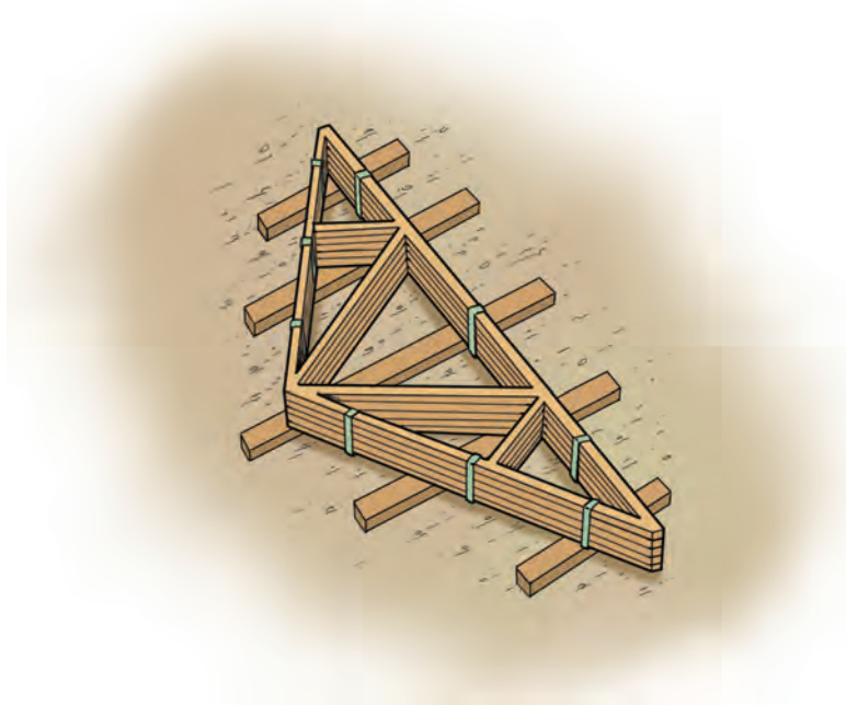
Figure 9.4. Stockage des fermes en position horizontale
