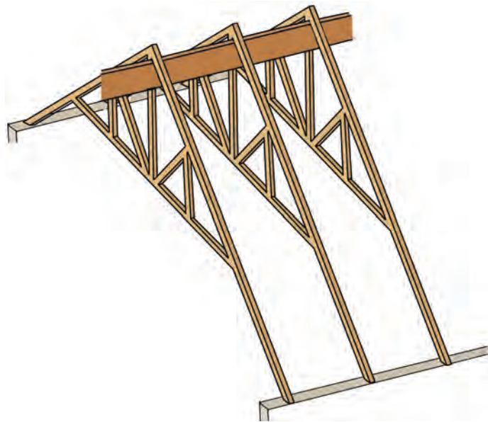
Figure 6.4.b. Stabilisation par une poutre longitudinale verticale
