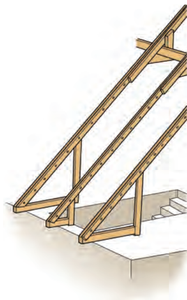
Figure 8.3. Renfort des pièces au voisinage d'une trémie d'escalier
