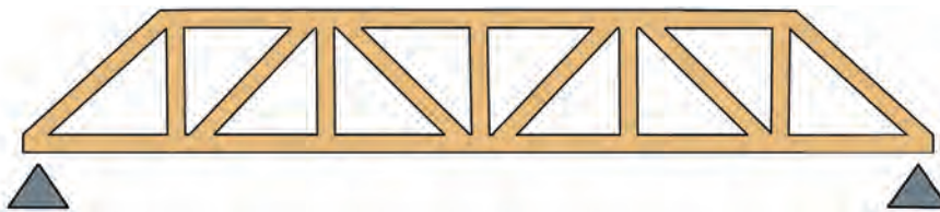
Figure 1.11. Fermes tronquées
