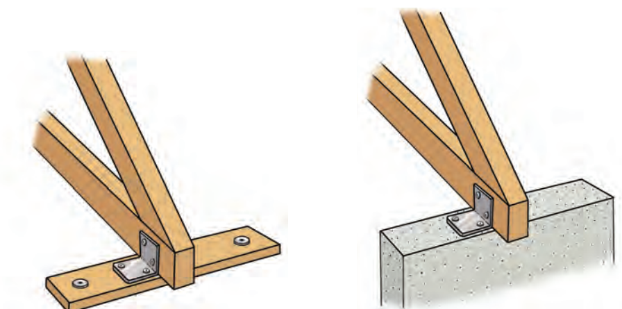
Fixation satisfaisante des fermes par équerres
