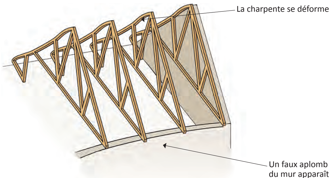
Figure 6.7. Déformation dissymétrique d'une ferme boiteuse
