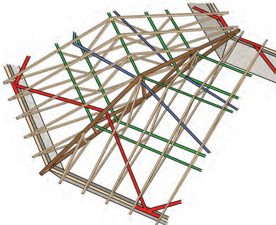
Figure 1.24. Exemple d'Arêtier-Noue
