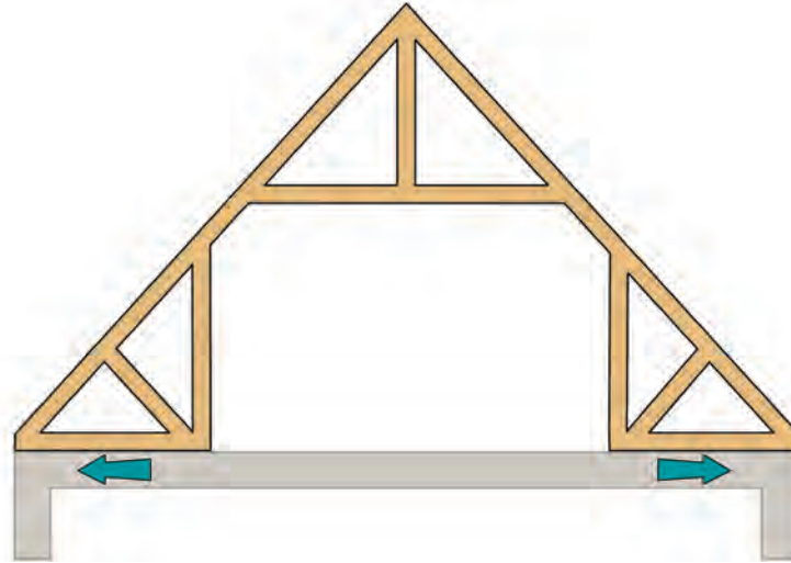
Figure 1.14. Ferme de combles habitables en « A »
