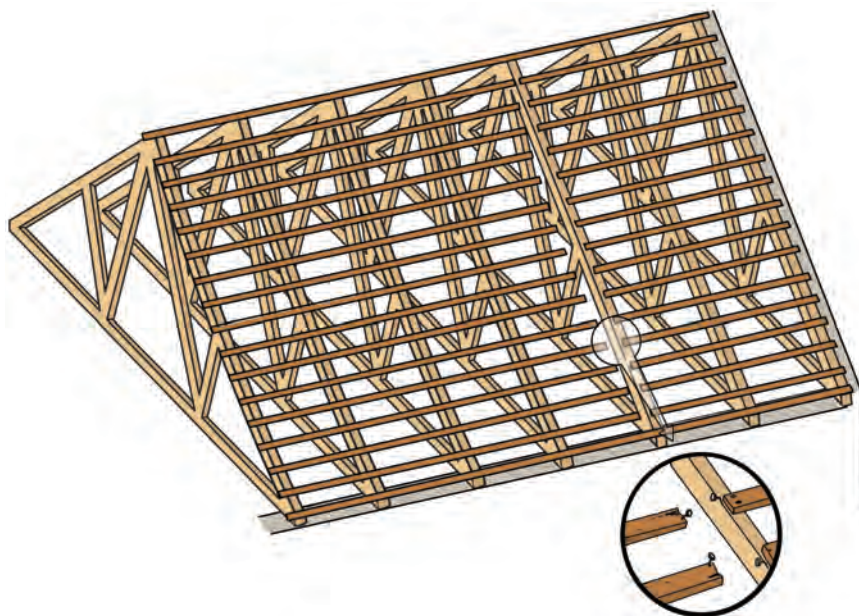
Figure 2.3. Déclouage des lisseaux assurant seuls le rôle d'antiflambement
