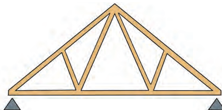
Figure 1.4. Ferme en « W » : La plus courante
