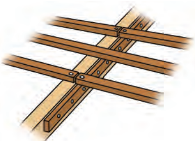
Figure 2.4. La bonne façon de clouer les lisseaux
