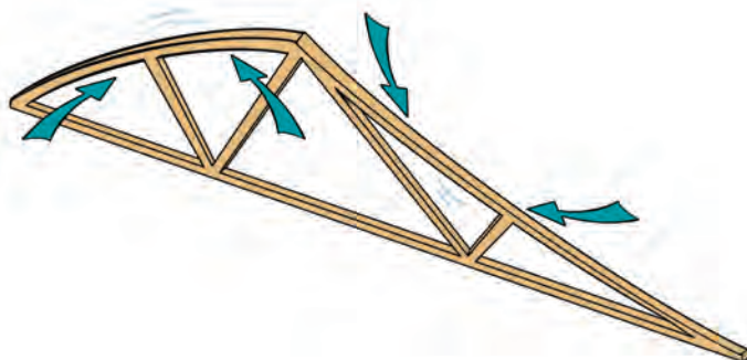
Figure 2.1. Flambement d'un arbalétrier – L'arbalétrier, comprimé, se déforme dans le sens de son épaisseur
